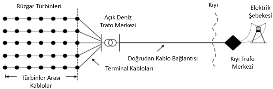
Şekil 5. Deniz Üstü RES'in Şebekeye Bağlanması (Üstten Görünüm)
