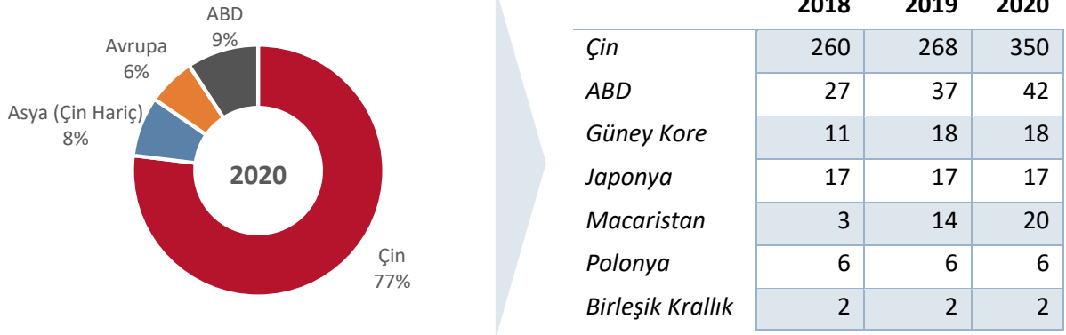
Grafik 3. Ülke Bazında Li-İyon Pil Üretim Kapasitesi (GWh/yıl)
