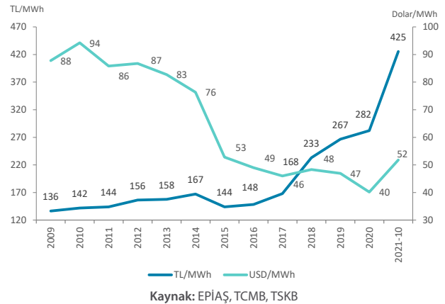
Grafik 13: Yıllık Ağırlıklı Ortalama PTF Gelişimi
