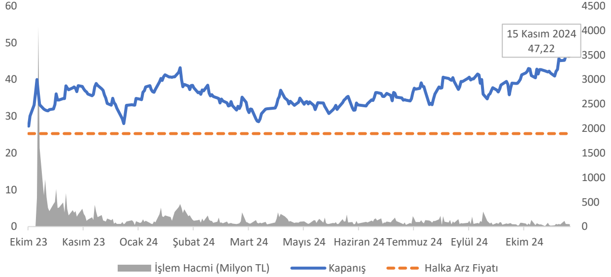
Grafik 1: Borlease Pay Fiyatı
