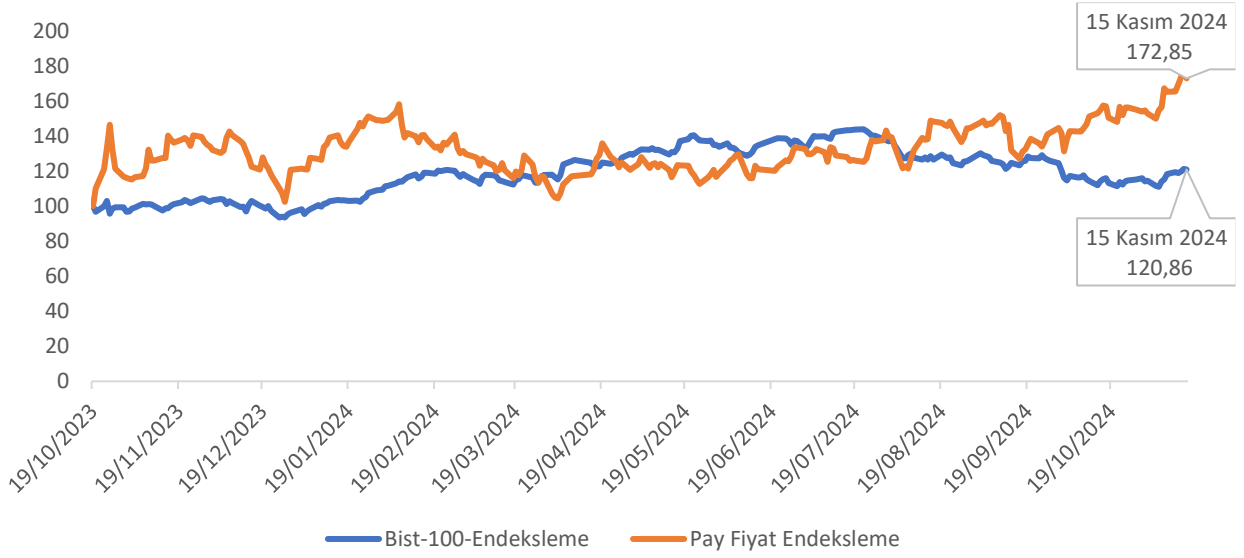
Grafik 3: BIST 100 Endeksi ve Borlease Otomotiv A.Ş.
